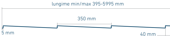
SECȚIUNE LOGITUDINALĂ
